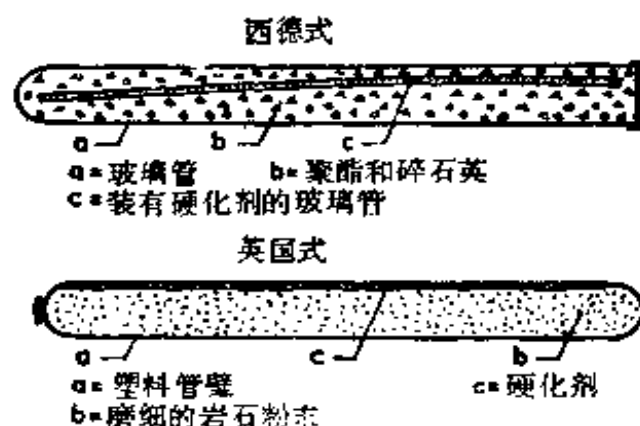
图 14 聚酯树脂筒
