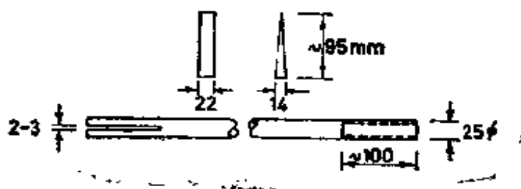
图 12 裂缝及楔块锚杆
