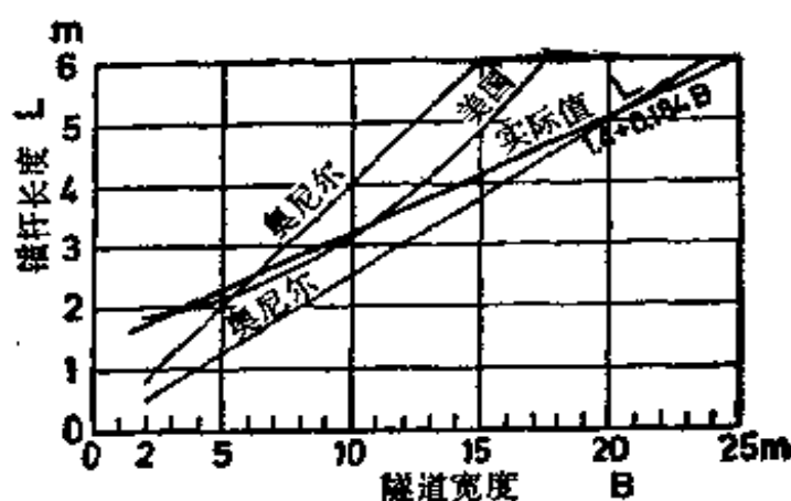
图 48 锚杆长度尺寸曲线
